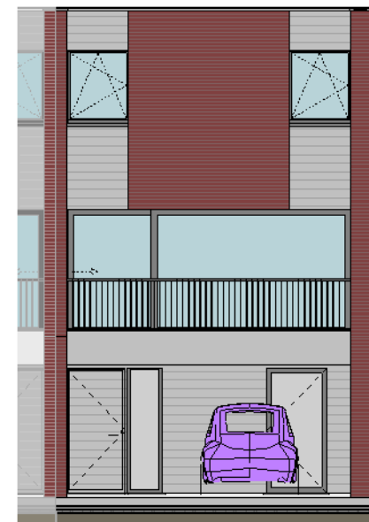
3 VOORGEVEL 1 : 50
