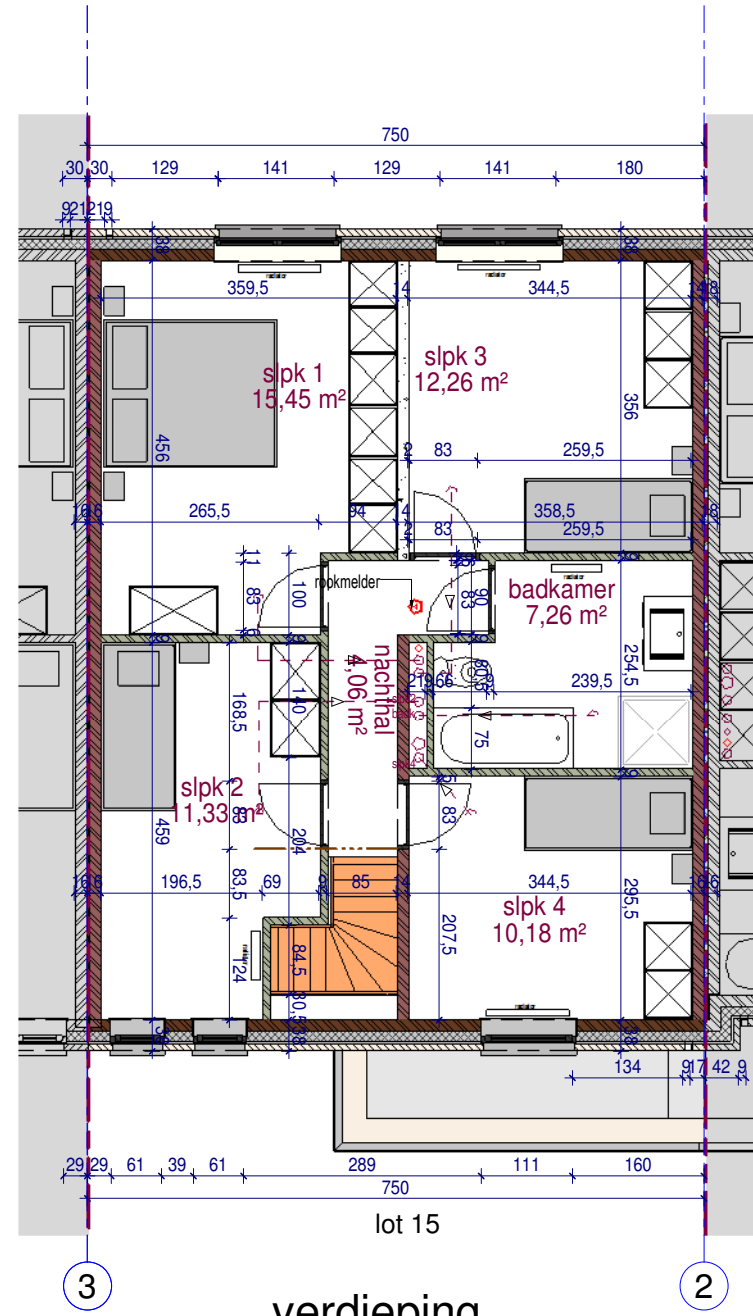
3 2 verdieping
