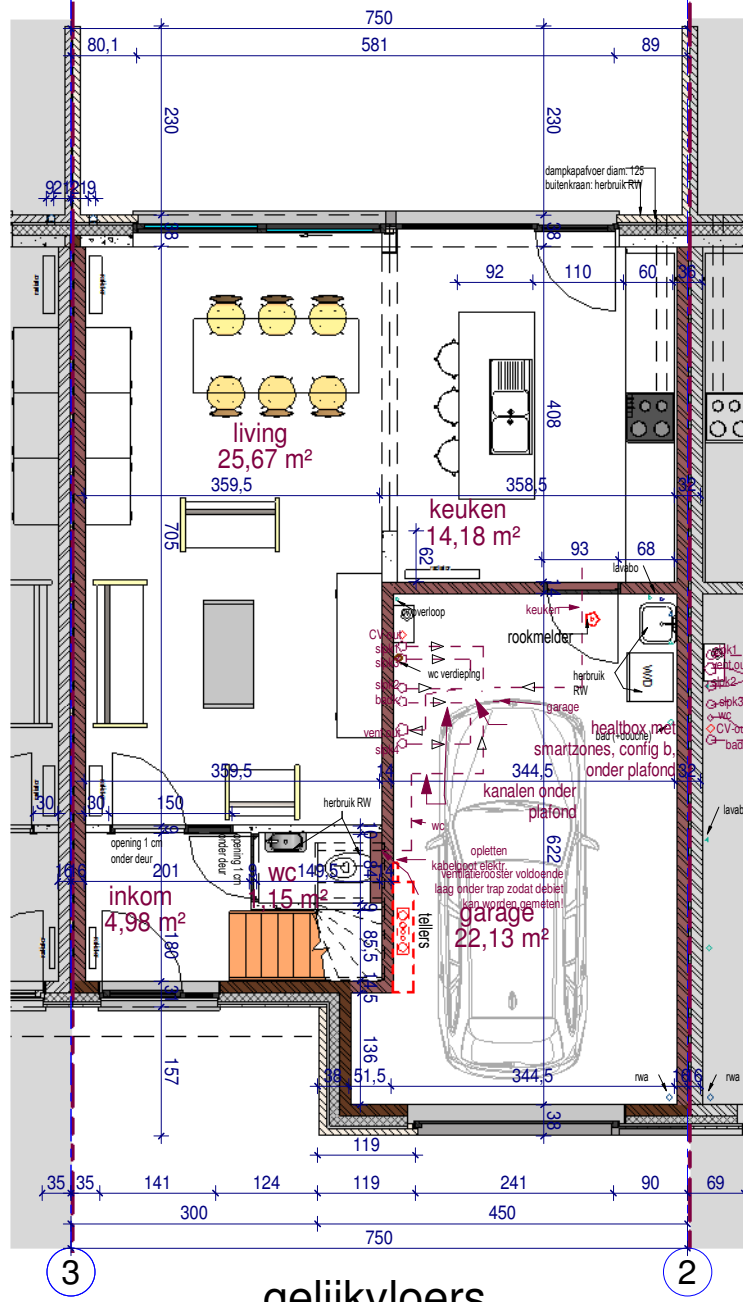
3 2 gelijkvloers
