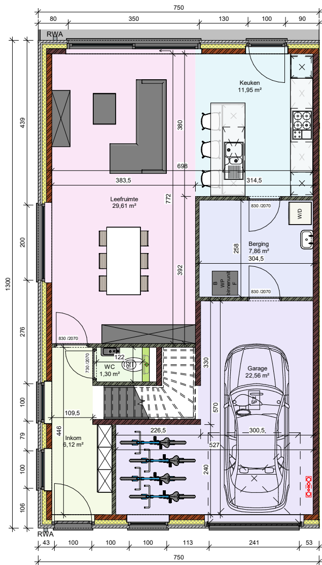
Gelijkvloers LL - lot 11
