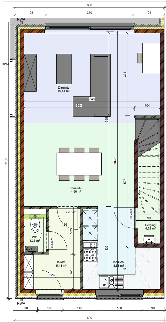
Gelijkvloers LL - lot 13
