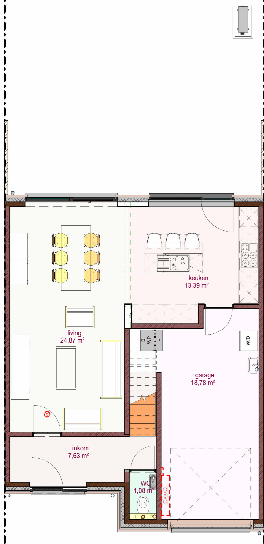
1 Gelijkvloers 171 LL 1 : 70
