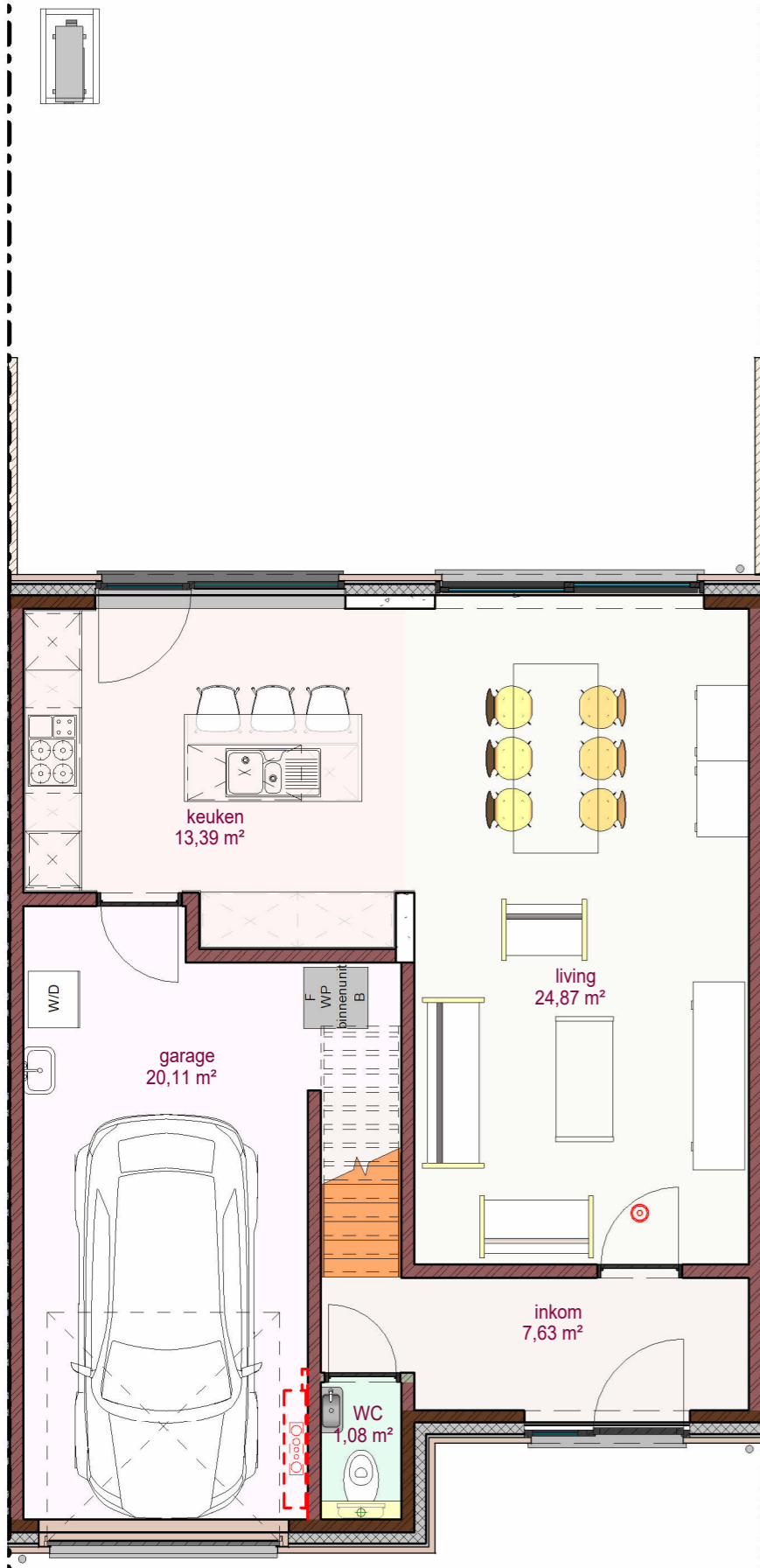
1 Gelijkvloers 174 LL 1 : 70
