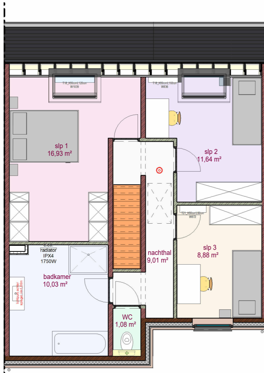
2 Verdieping 174 LL 1 : 70
