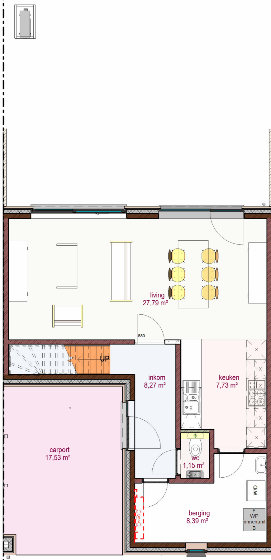
1 Gelijkvloers 176 LL 1 : 70
