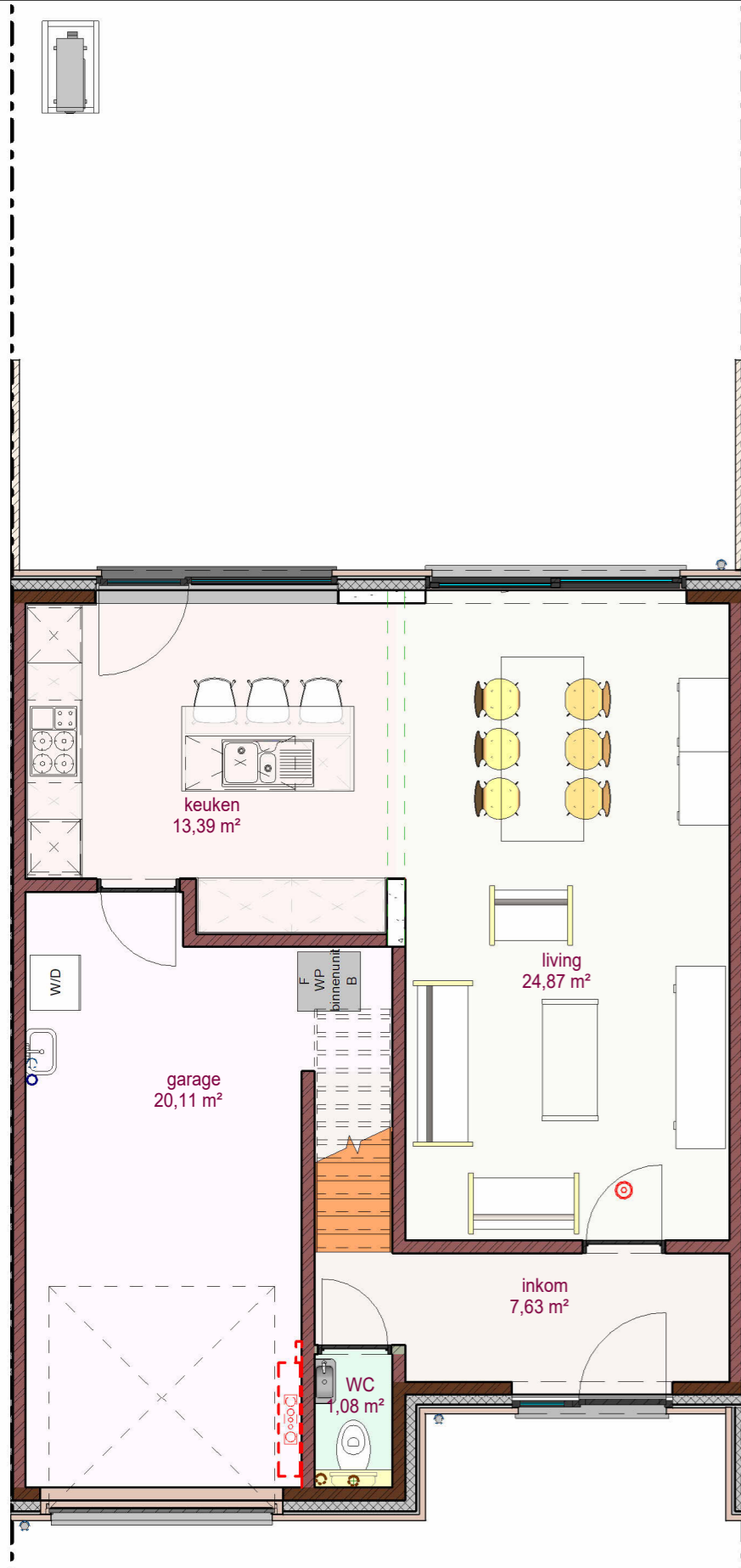
1 Gelijkvloers 181 LL 1 : 70
