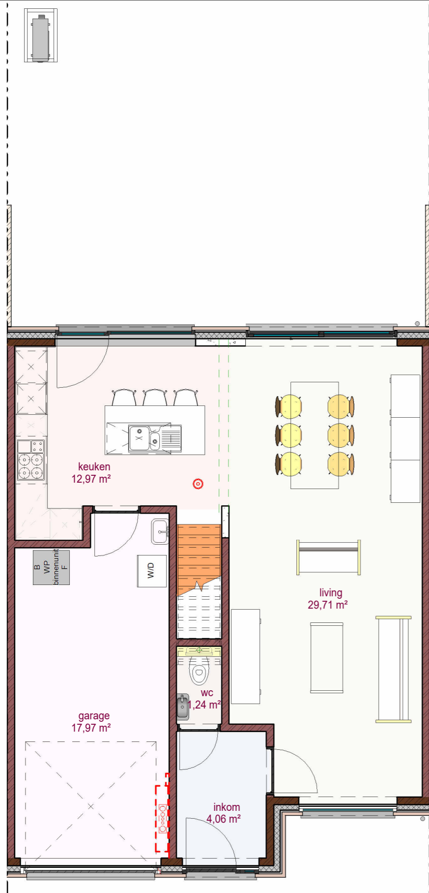
1 Gelijkvloers 183 LL 1 : 70
