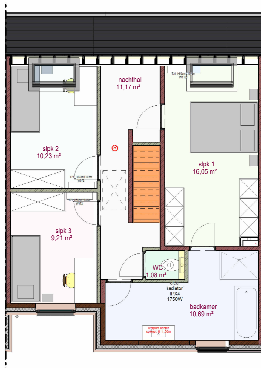
2 Verdieping 184 LL 1 : 70
