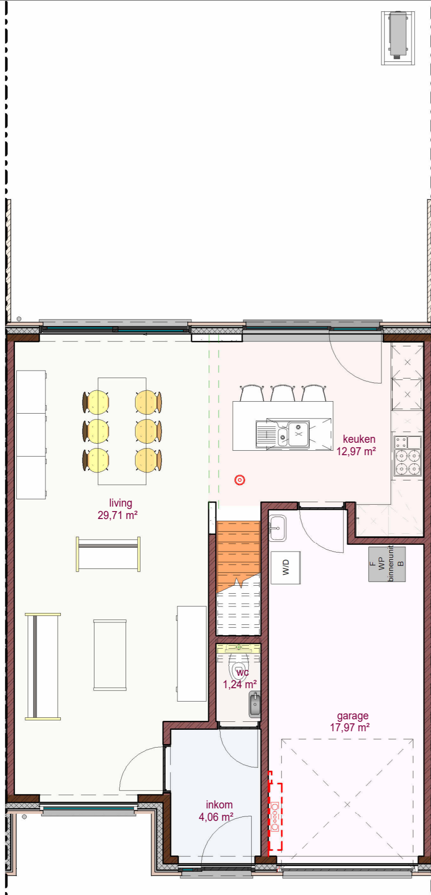
1 Gelijkvloers 184 LL 1 : 70
