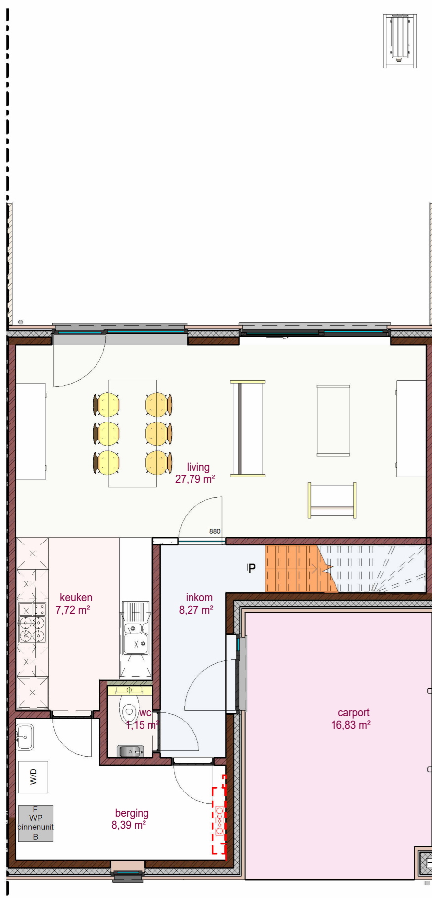
1 Gelijkvloers 186 LL 1 : 70
