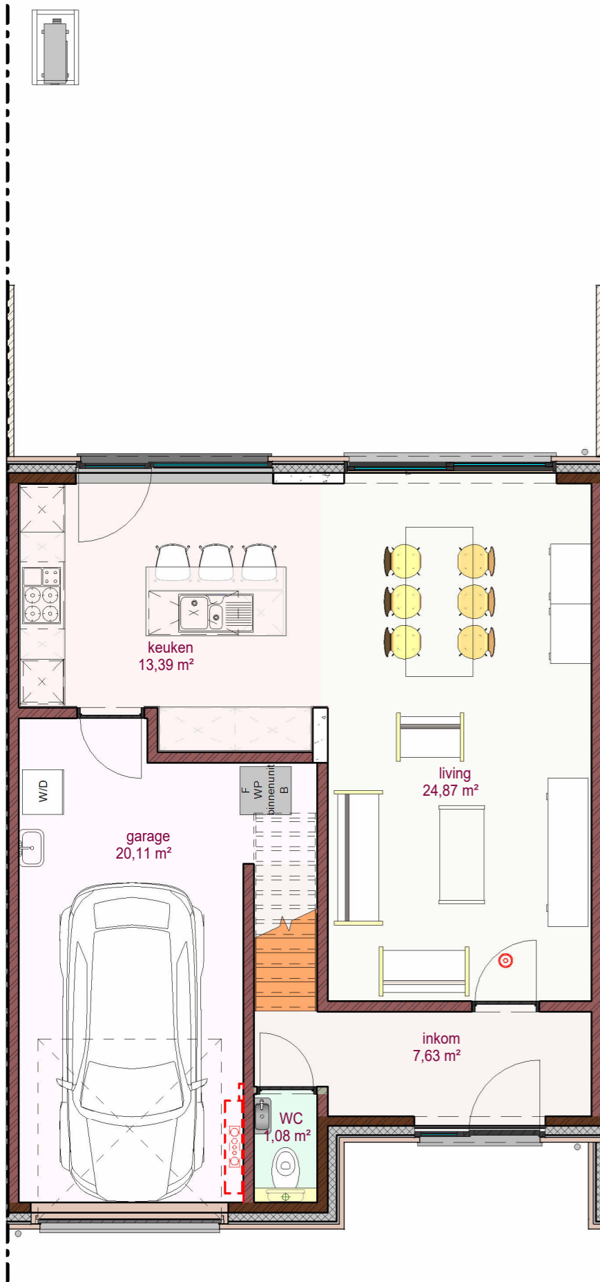
1 Gelijkvloers 187 LL 1 : 70
