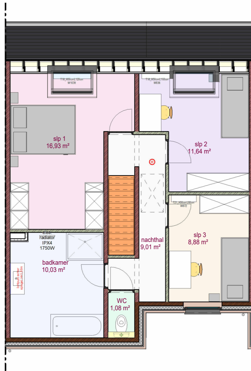
2 Verdieping 187 LL 1 : 70
