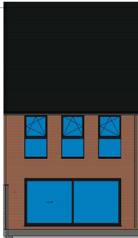
3 achtergevel - lot 11 LL 1 : 65
