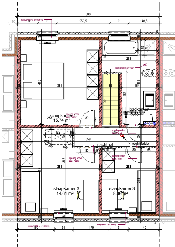
1ste verdieping
