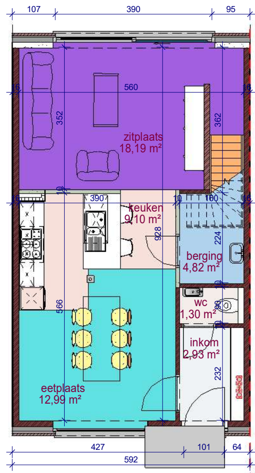
Lot 18 gelijkvloers
