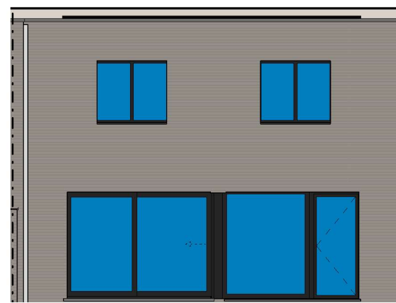
Achtergevel lot 198
