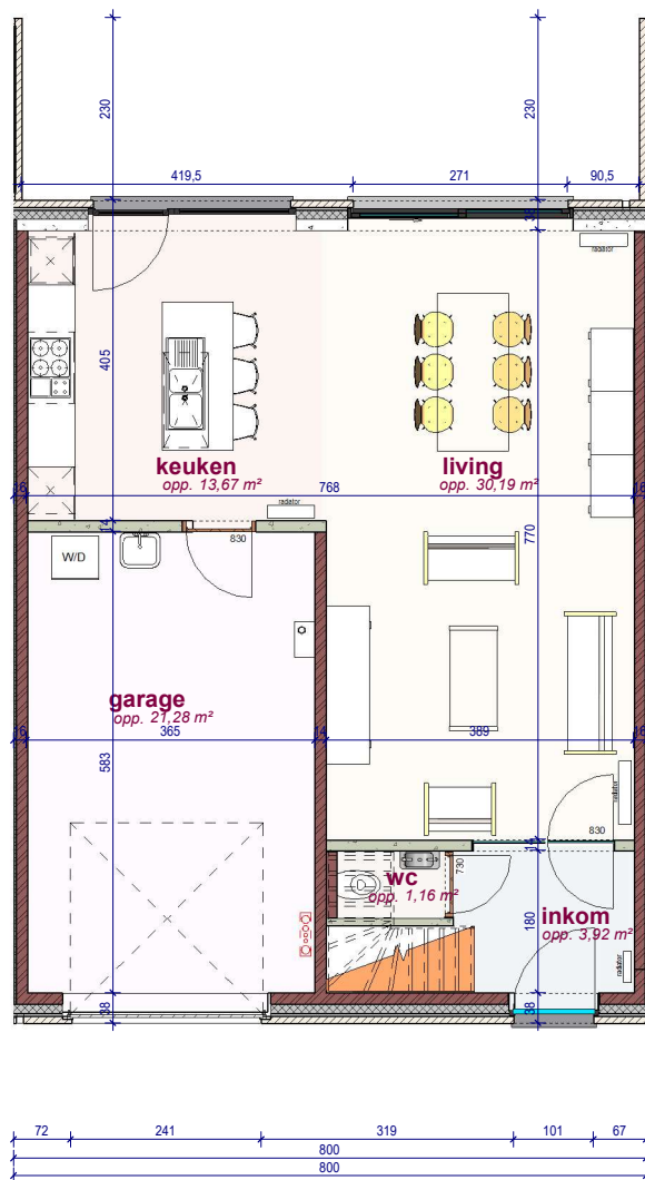
gelijkvloers lot 200 LL
