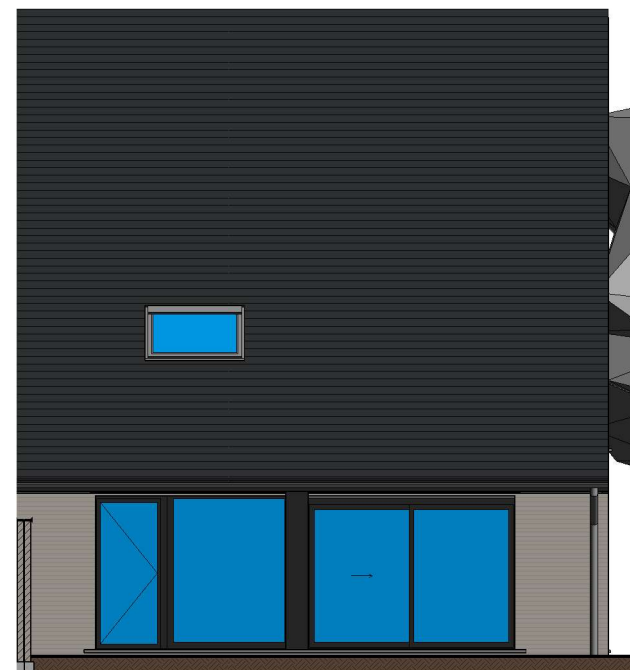
Achtergevel lot 210
