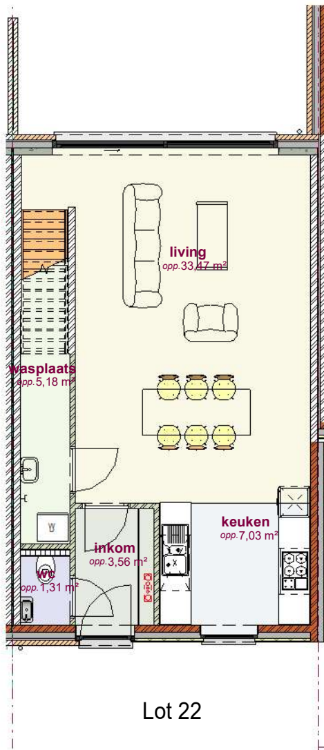
gelijkvloers - lot 22 LL
