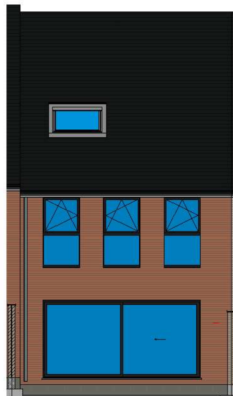
2 achtergevel - lot 22 LL 1 : 65
