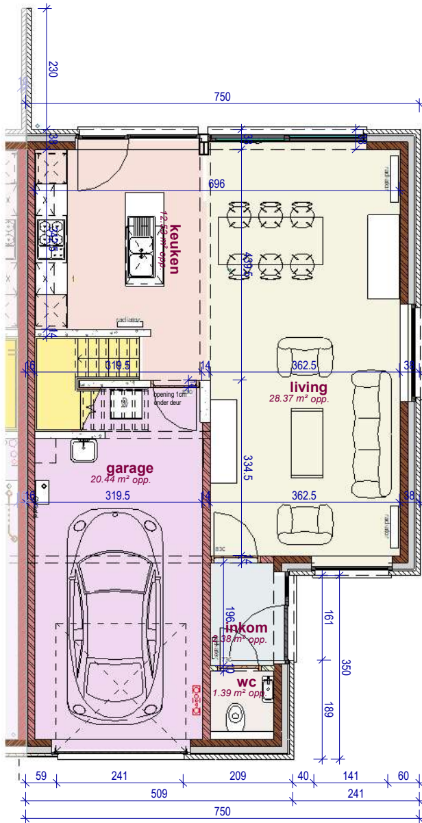
gelijkvloers 28 LL
