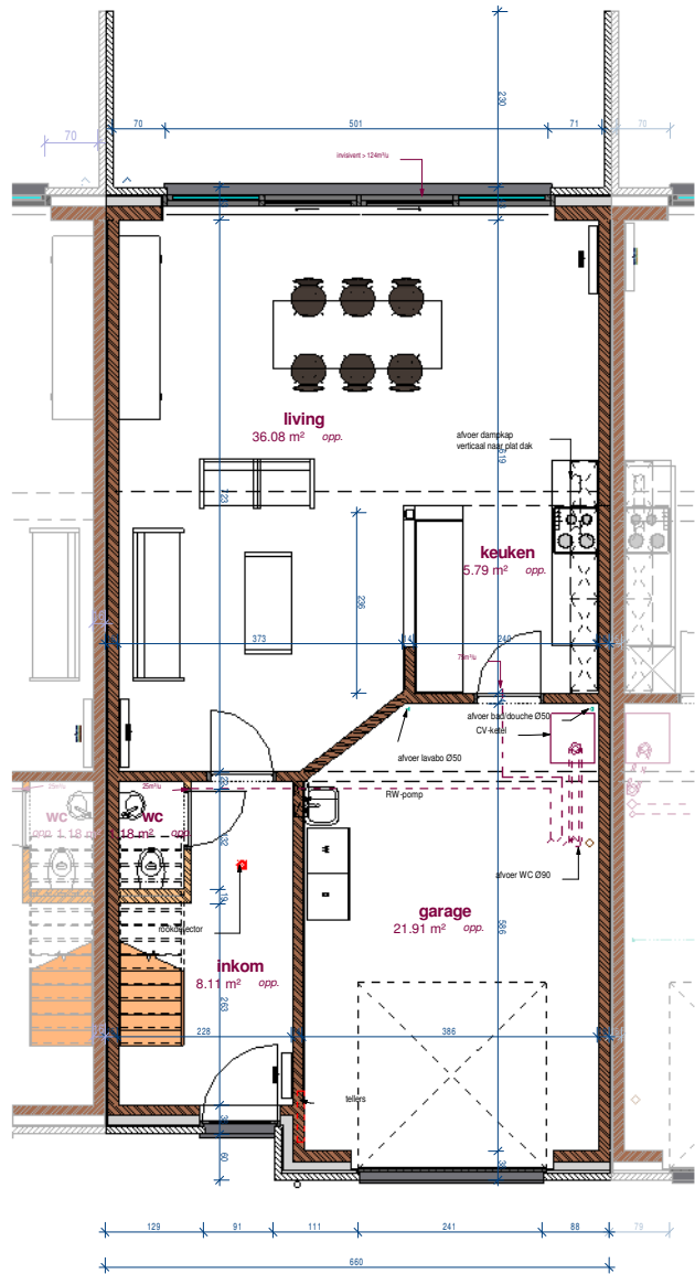
gelijkvloers
