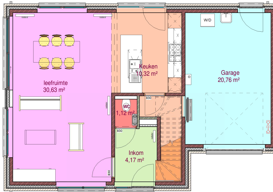
1 gelijkvloers woning 6 LL 1 : 75
