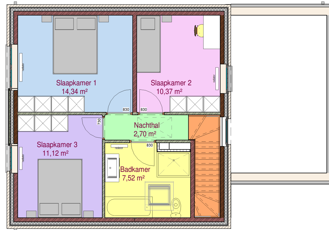
2 verdieping woning 6 LL 1 : 75
