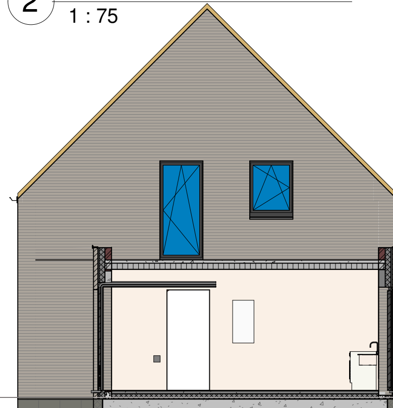
4 zijgevel rechts woning 6 1 : 75
