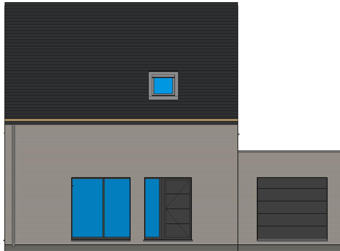
1 voorgevel woning 6 1 : 75
