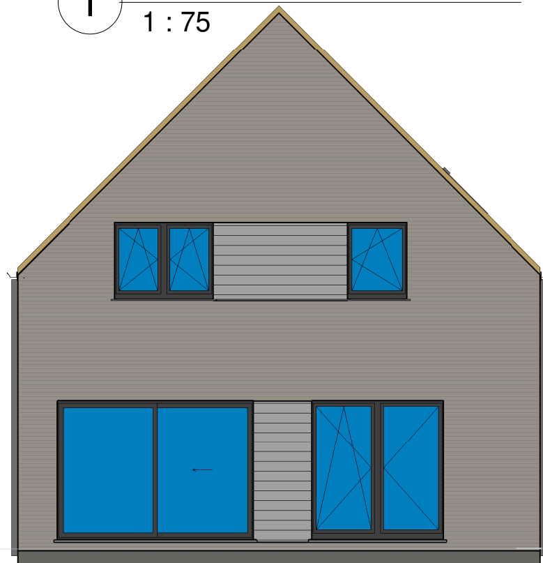
3 zijgevel links woning 6 1 : 75
