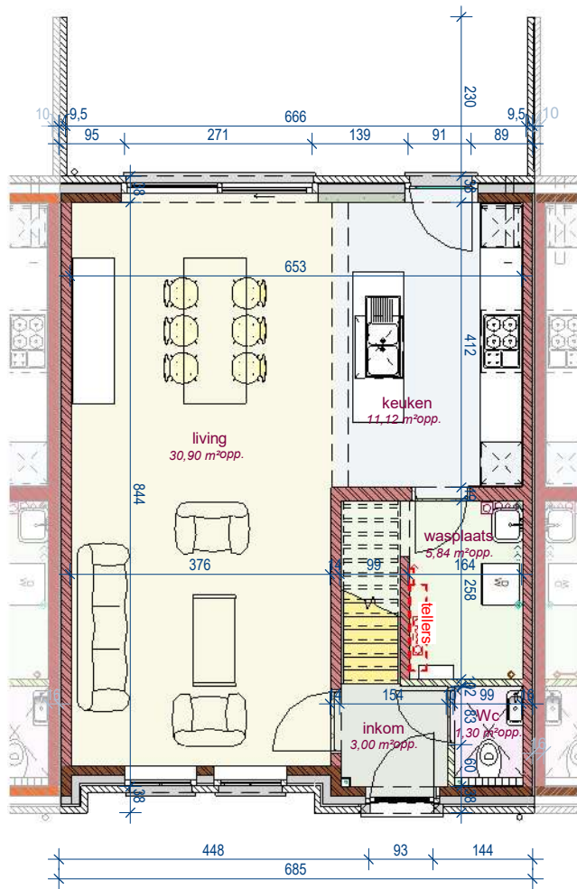
lot B6 gelijkvloers
