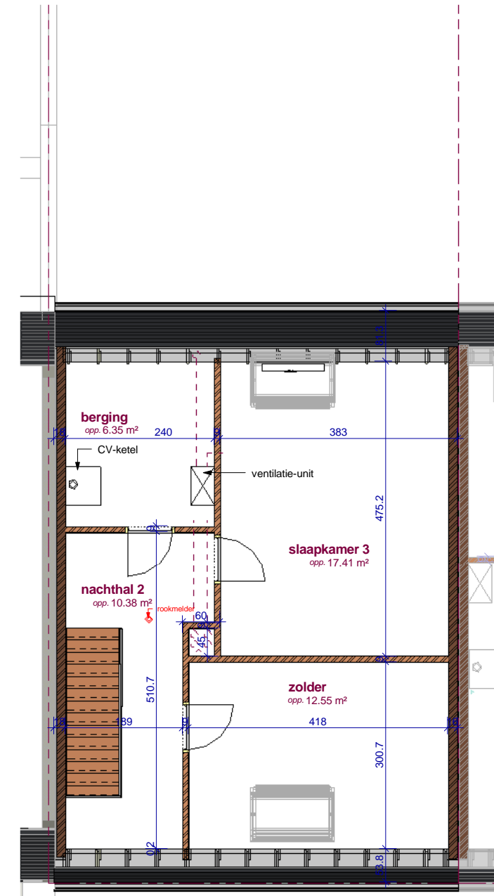
3 2de VERDIEPING 1 : 50
