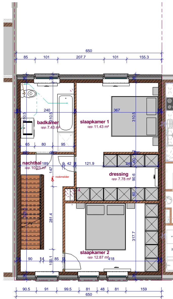
2 1ste VERDIEPING 1 : 50
