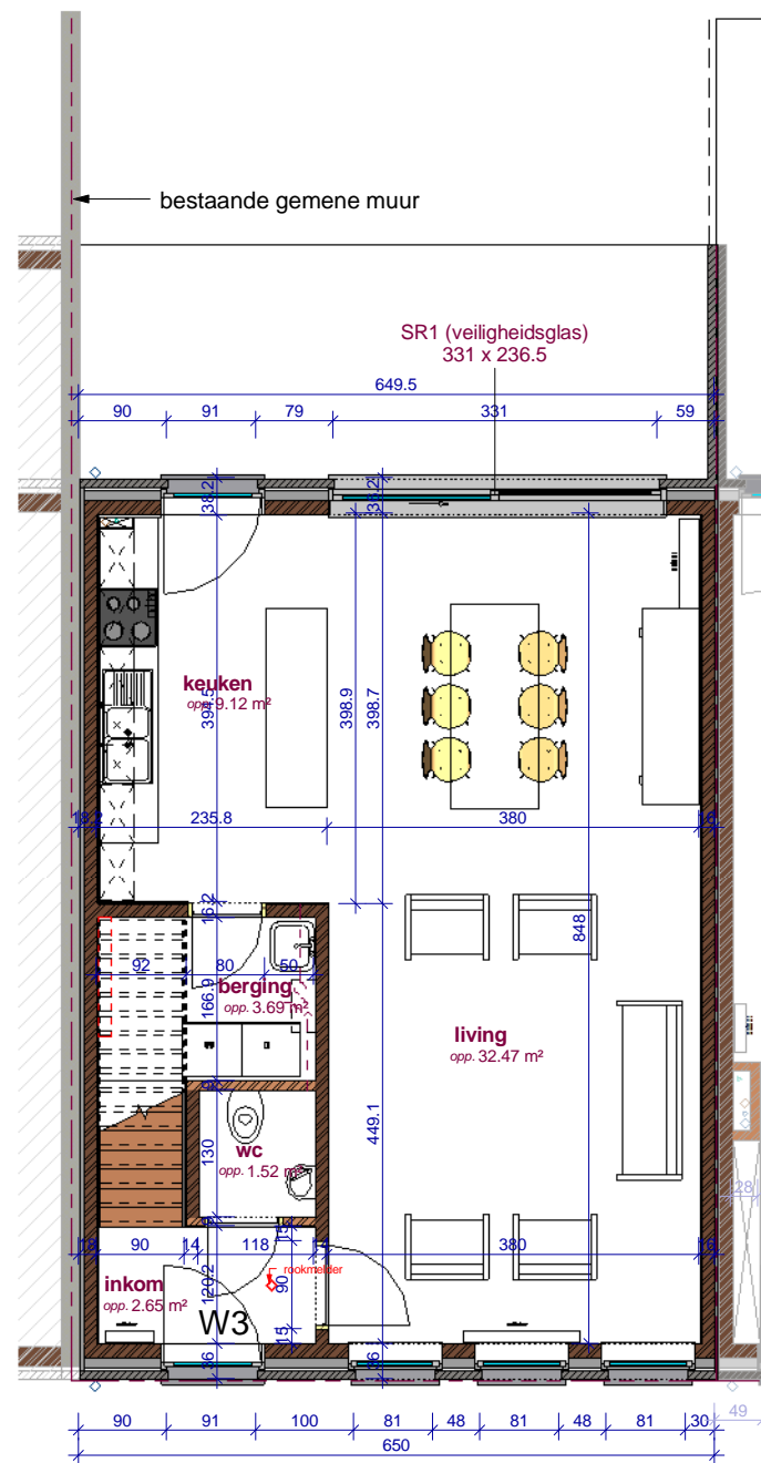
1 GRONDPLAN 1 : 50
